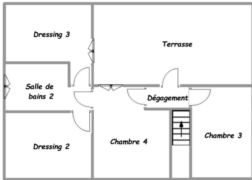
1er étage
